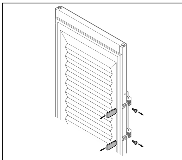
Fig. 24 Ispunjena vrata*
