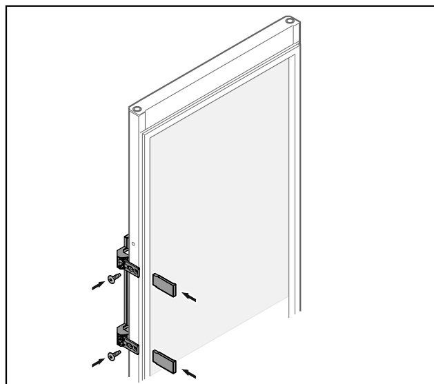
Fig. 28 Staklena vrata*
