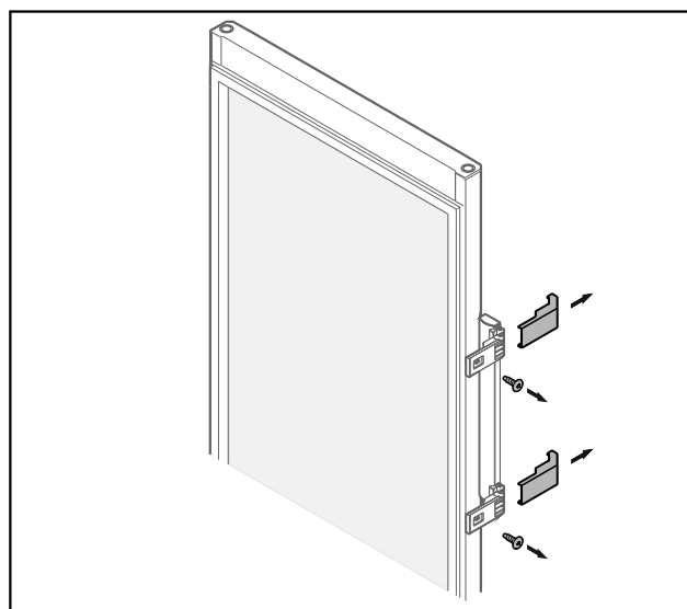
Fig. 25 Staklena vrata*
